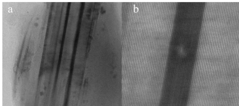
Rys. 12 Obrazy TEM i HRTEM CNT otrzymane z paku węglowego z dodatkiem nanocząstek ceramicznych.
