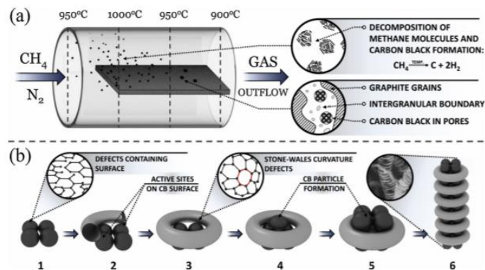
Rys. 6 Schemat przedstawiający wzrost toroidalnych nanorurek węglowych
