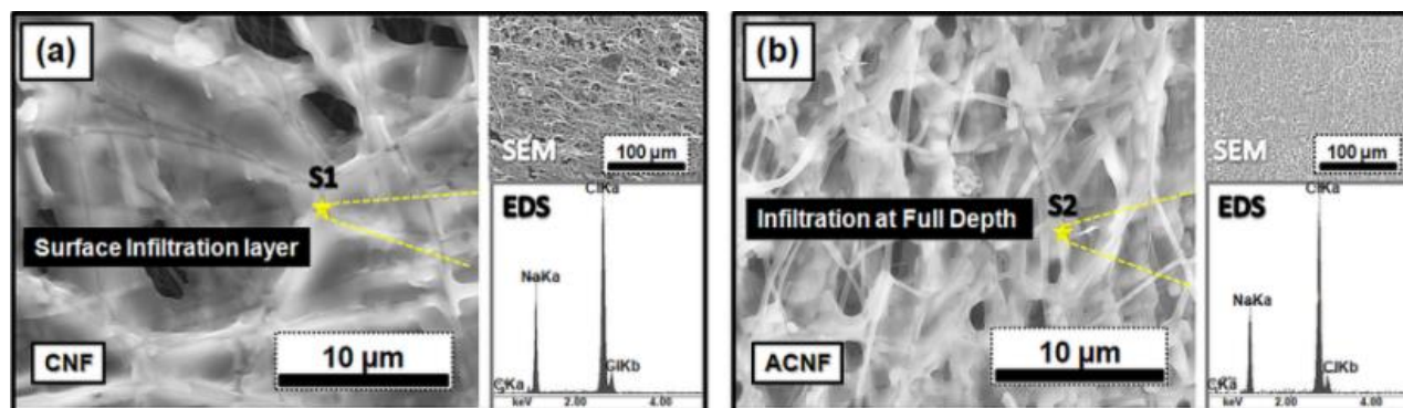
Rys. 1 Obrazy SEM i analizy EDS depozytu NaCl na powierzchni a) CNFs, b) ACNFs.
