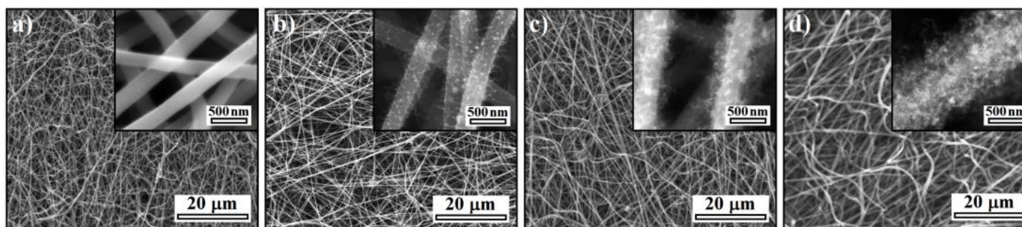
Rys. 2 Obrazy SEM nanokompozytów hierarchicznych eCNF/dCNT, zawierających odpowiednio 0% (a), 1,5% (b), 3% (c) i 4,5% (d) \text{Fe}(\text{Acac})_3 .
