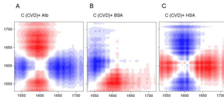
Rys. 11 Asynchroniczne widma ramanowskie próbek węglowych inkubowanych różnymi rodzajami albumin
