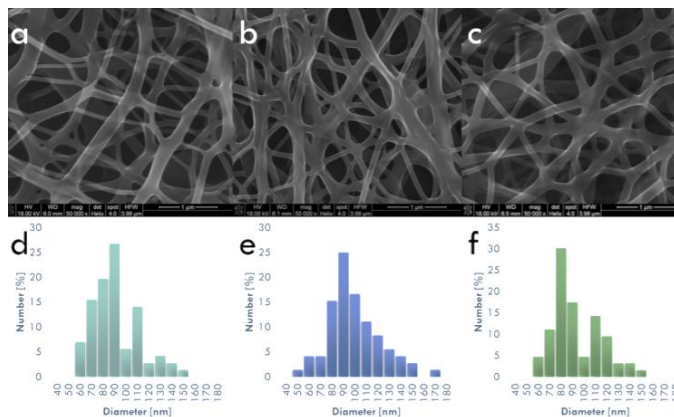
Rys. 9 Obrazy SEM nanowłókien węglowych i rozkłady wielkości średnic.
