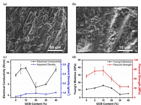
Rys. 13 Obrazy SEM nanokompozytu przewodzącego: żywica epoksydowa + rCF + sadza grafityzowana oraz wyniki badań elektrycznych i mechanicznych tych próbek.
