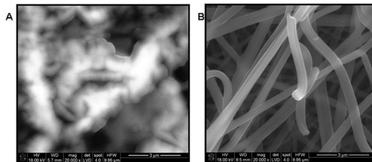
Rys. 14 Warstwa nanometryczna z albumin otrzymana na: MWCNTs nanoszonych metodą EPD(A), nanowłóknach węglowych CNF (B).
