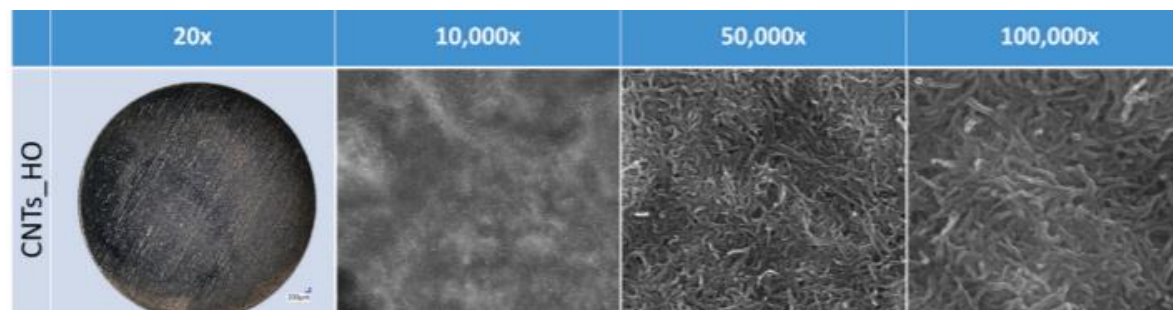
Rys. 3 Obrazy mikroskopowe warstw z nanorurek węglowych przy różnym powiększeniu.
